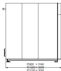
Vaizdas iš šono FS 800, 1000, 1200
